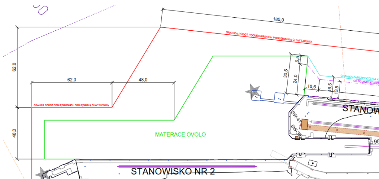
Rys. Zakres umocnienia dennego przy Stanowisku nr 2 TPŚ
