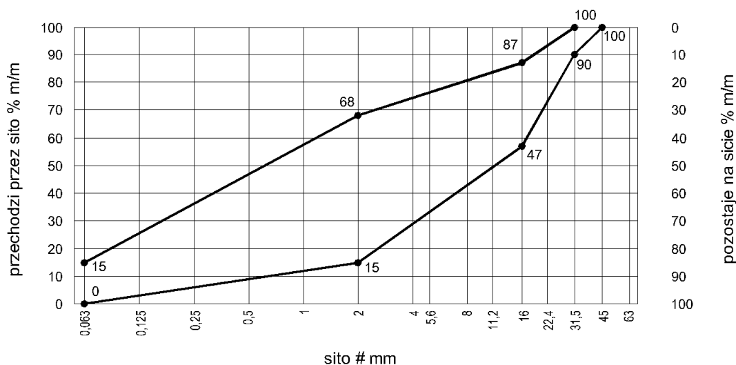
Rysunek 1. Obszar uziarnienia optymalnych mieszanki żwirowych 0/31,5 mm
