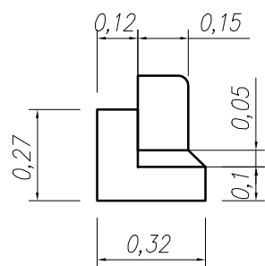
krawężnik najazdowy 15x22 cm
