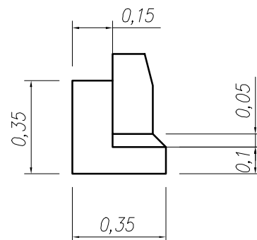
krawężnik betonowy 15 x 30 cm
