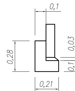
obrzeże betonowe 8x30 cm
