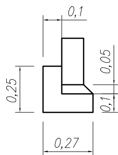
opornik betonowy 12 x 25 cm
