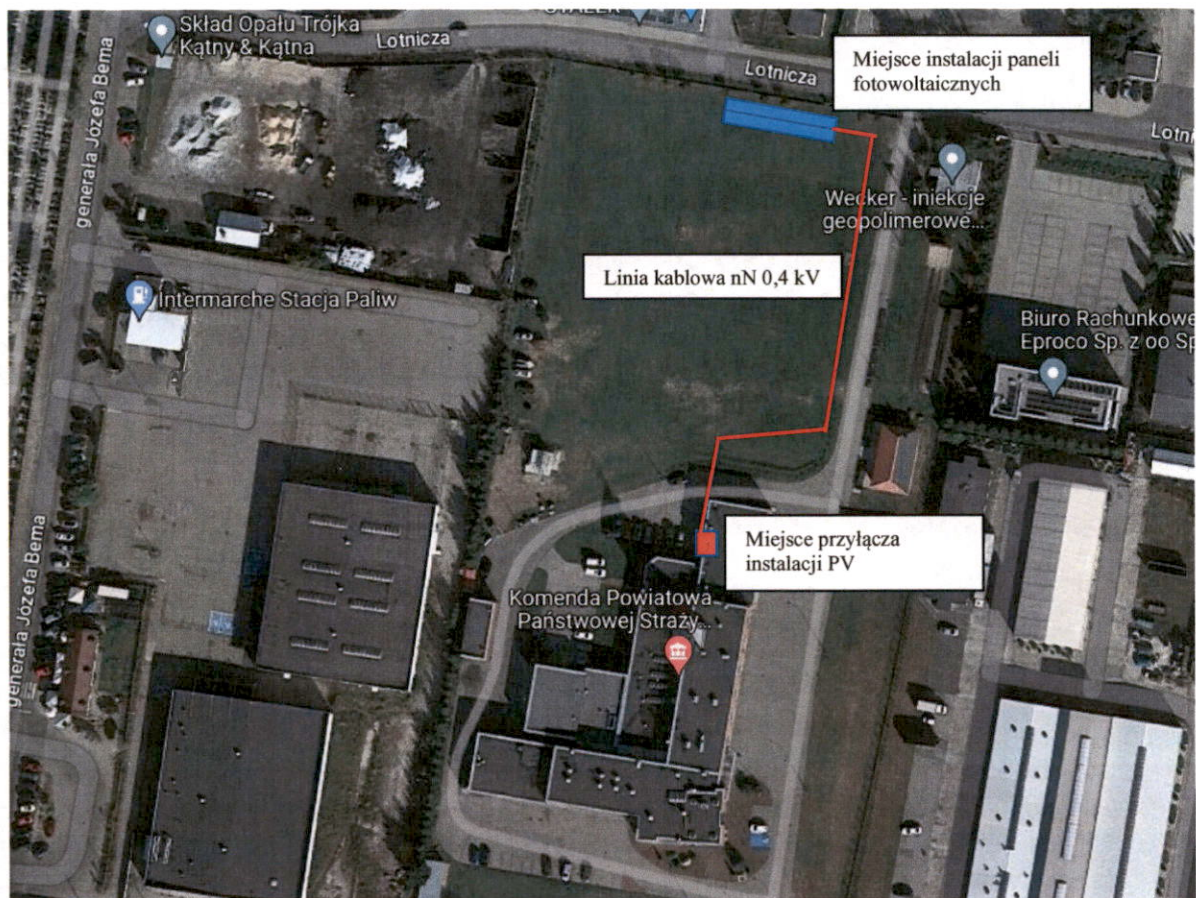
Rys.1 Obiekt KP PSP w Ostrowie Wielkopolskim z zaznaczonym miejscem planowanego montażu paneli fotowoltaicznych.
